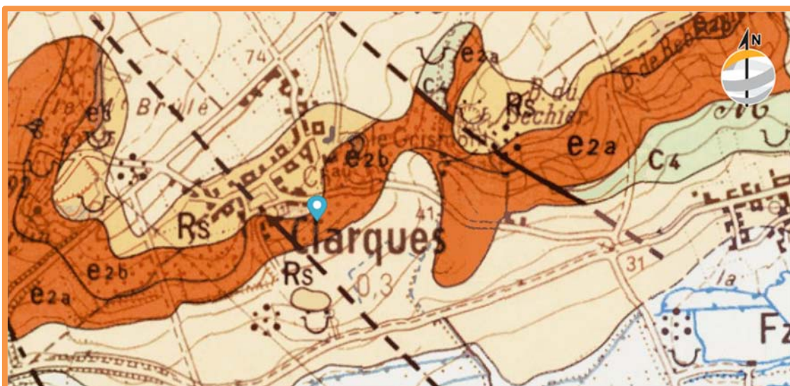
Extrait de la carte géologique du BRGM
