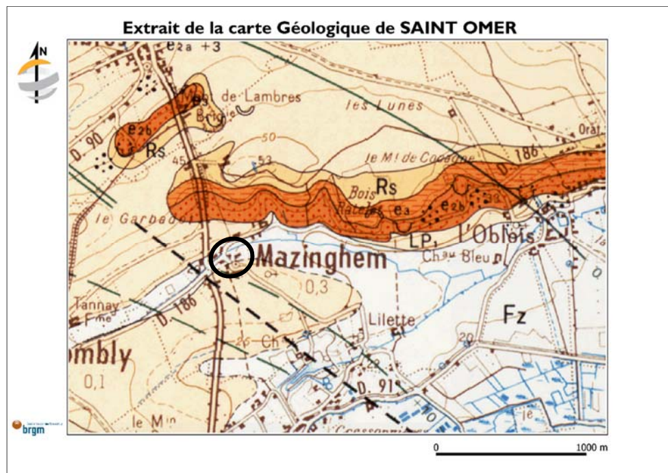
Extrait de la carte géologique de SAINT-OMER
