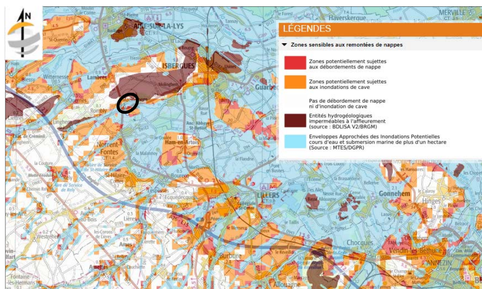
Extrait de la carte de l'aléa remontée de nappe-inondation
