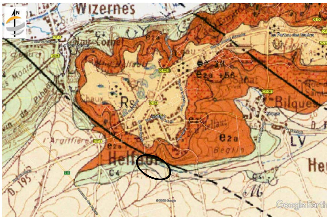
Extrait de la carte géologique de SAINT OMER
